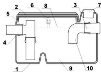
Принципиальная схема жиρούловителя серии СЖ "Оптимa"
