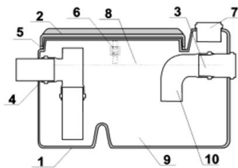
Принципиальная схема жируловителя серии СЖ "Оптимa"
