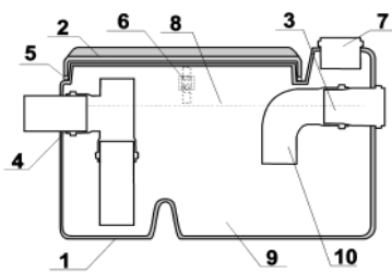
Принципіальна схема жиросилоуловителя серії СЖ "Оптима"
