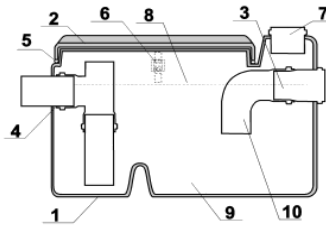
Принципова схема жировловлювача серії СЖ "Оптіма"
