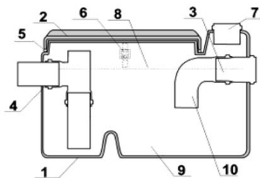
Принципальная схема жируловителя серии СЖ "Оптима"
